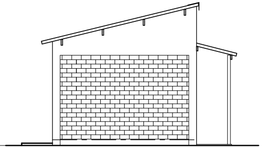
ELEVATION 4
