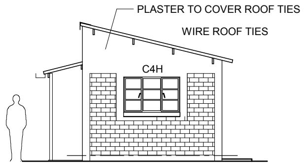
ELEVATION 2
