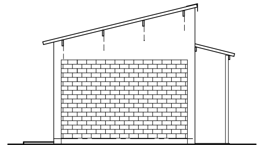
ELEVATION 4
