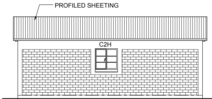
ELEVATION 3
