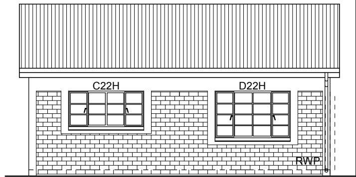
ELEVATION 3
