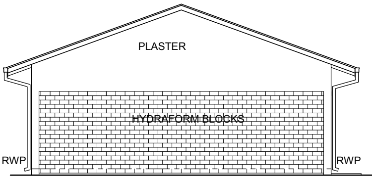
ELEVATION 4
