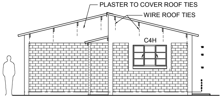
ELEVATION 2
