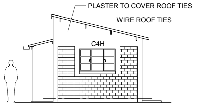
ELEVATION 2
